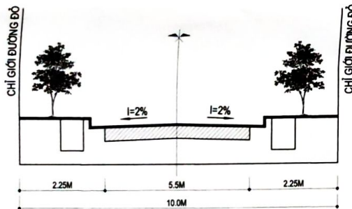
MẶT CẮT 1-1
