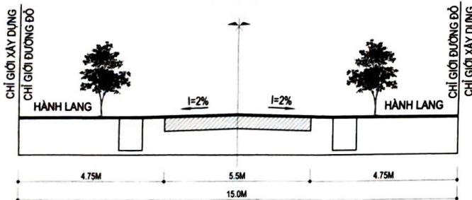
MẶT CẮT 2-2
